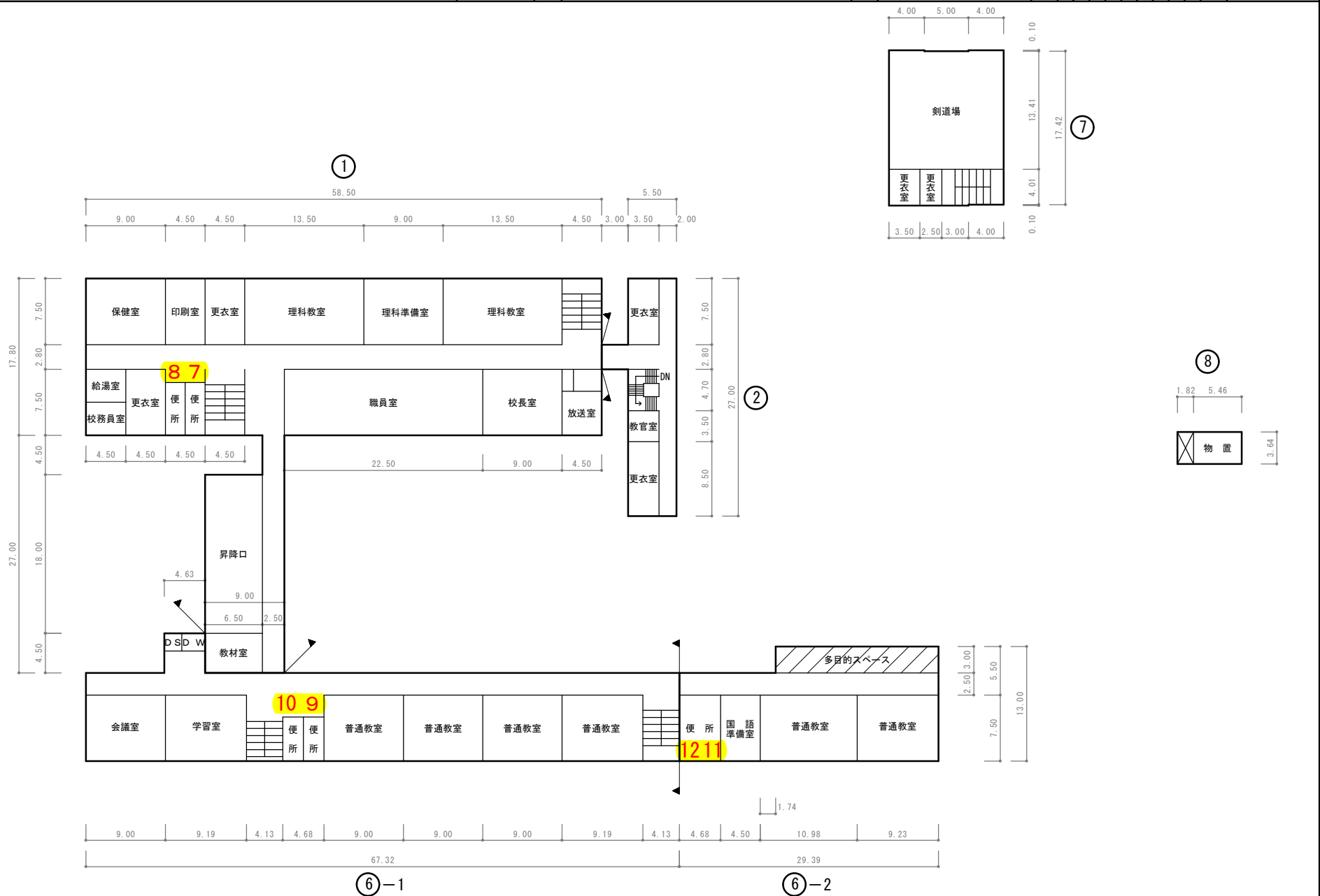
2階平面図
