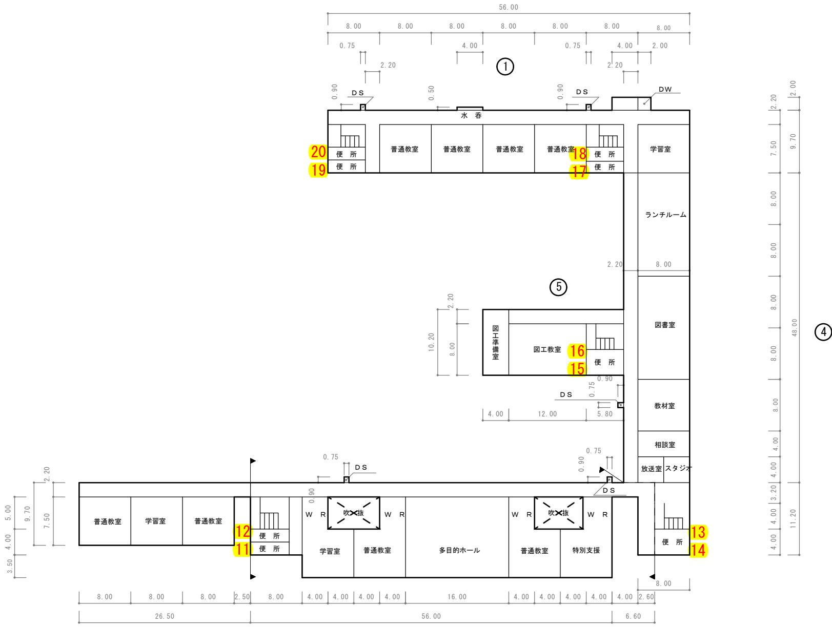
2 階 平 面 図
