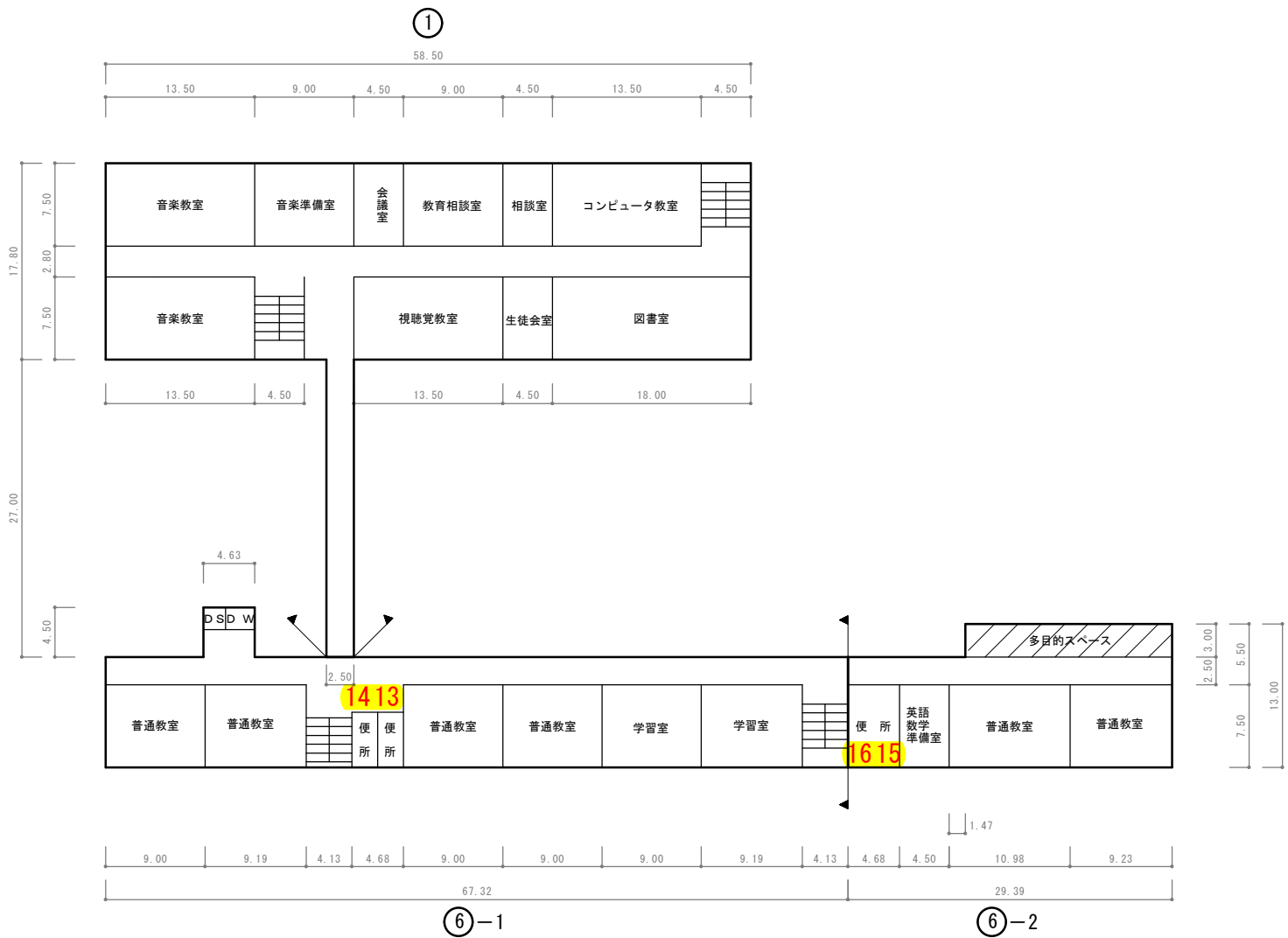
3 階 平 面 図
