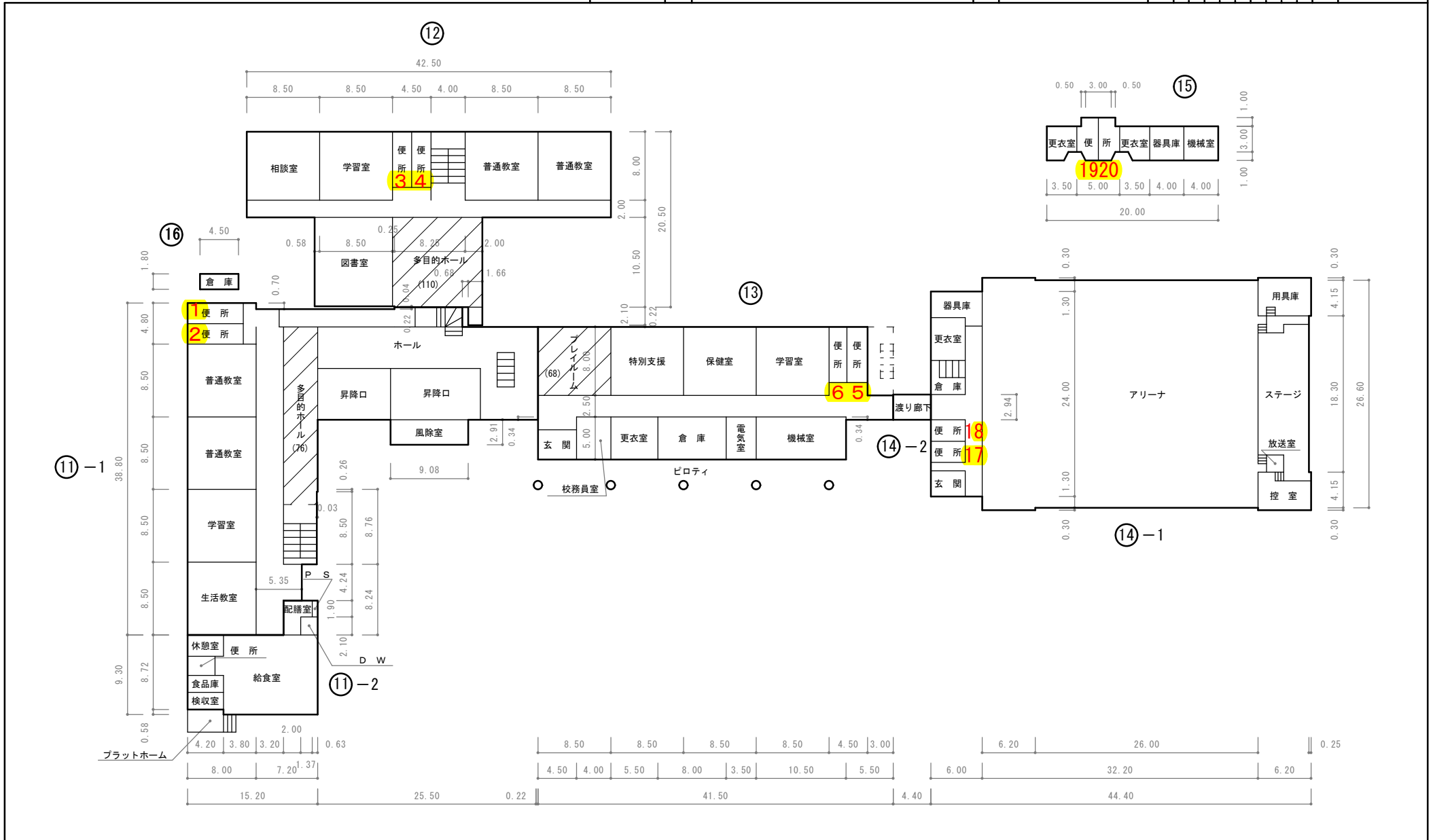
1 階 平 面 図
