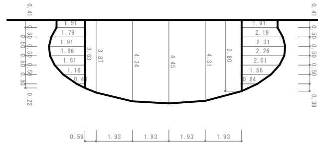
別図A 1/200
