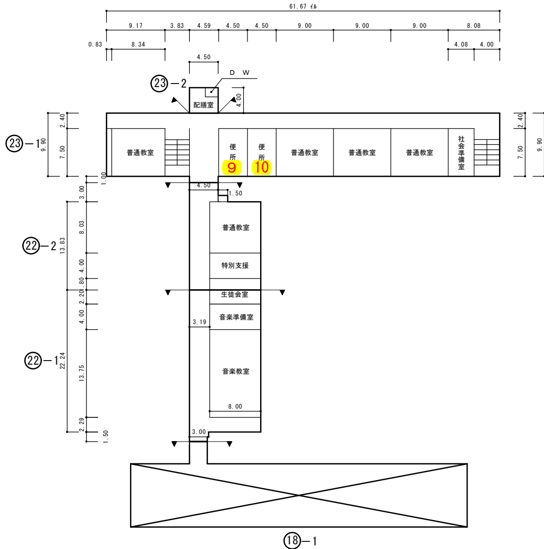
4 階 平面 図
