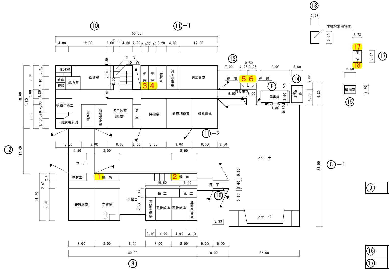
1 階 平 面 図
