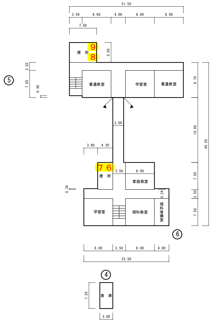
2 階 平 面 図
