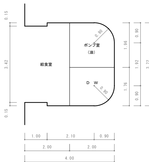
地階
