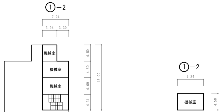
塔屋 2 階
