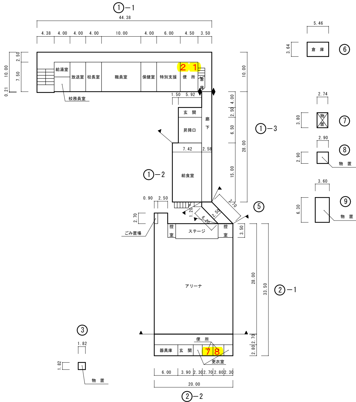
1 階 平 面 図
