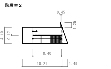
4 階 平 面 図
