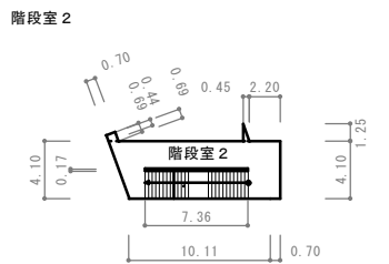
3 階 平 面 図
