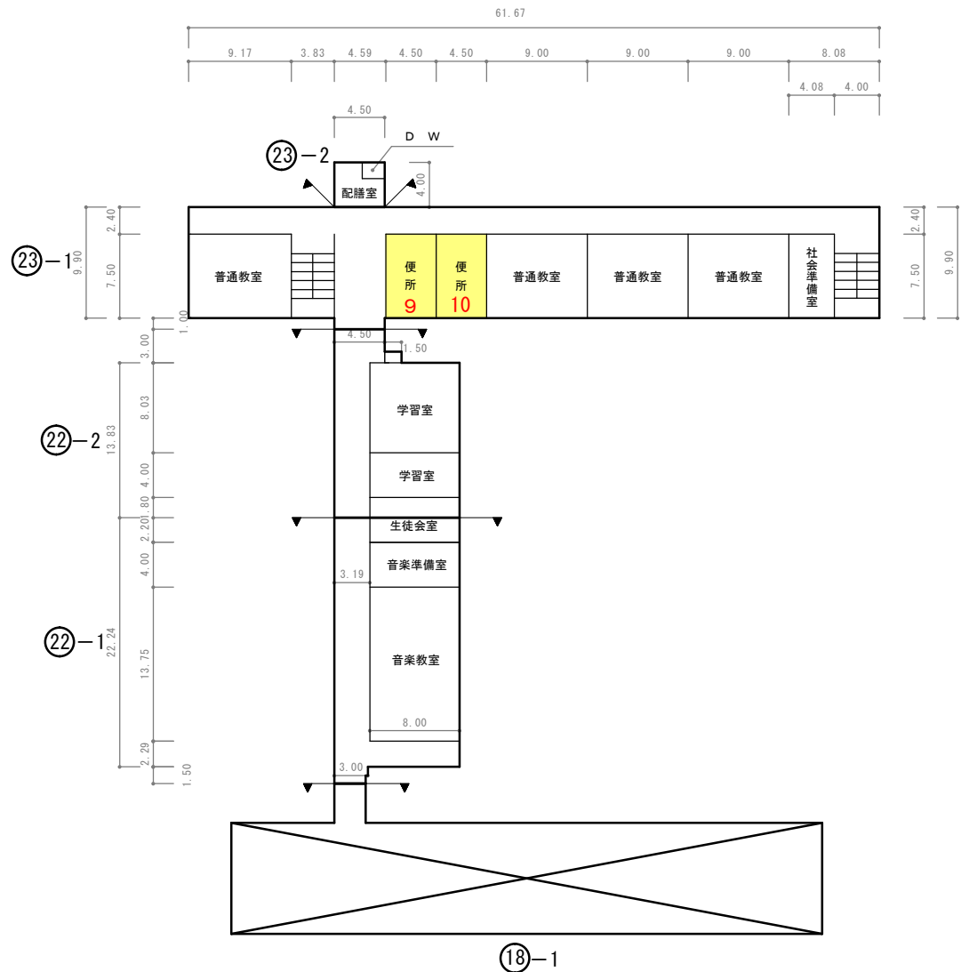
4 階 平面 図
