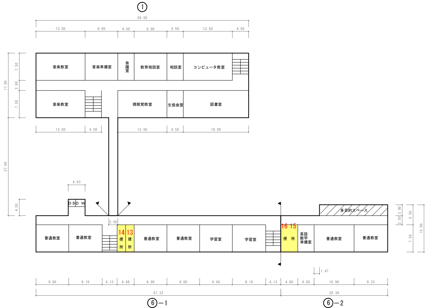
3 階 平 面 図
