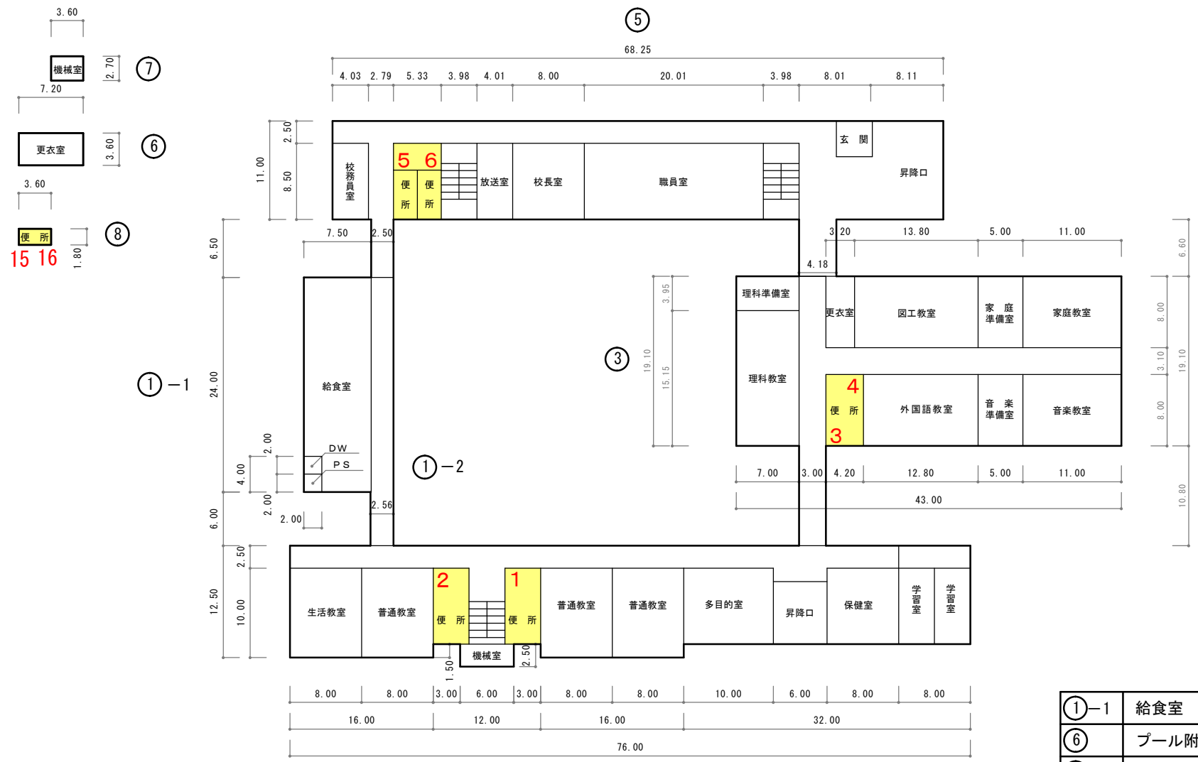
1 階 平 面 図
