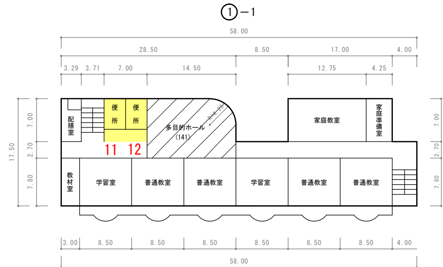
教室棟3階平面図
