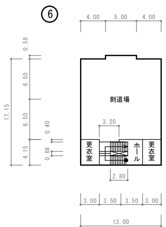
2階平面図
