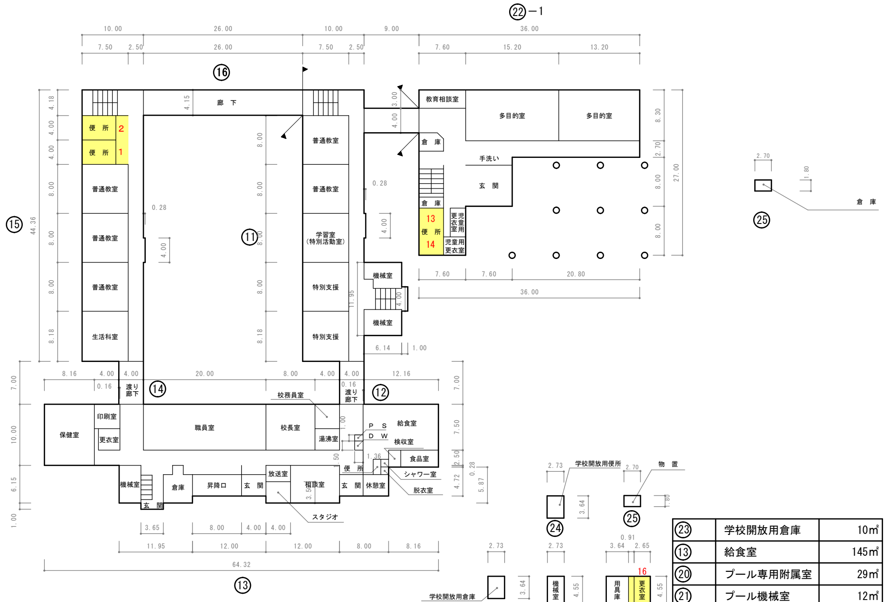
1 階 平 面 図
