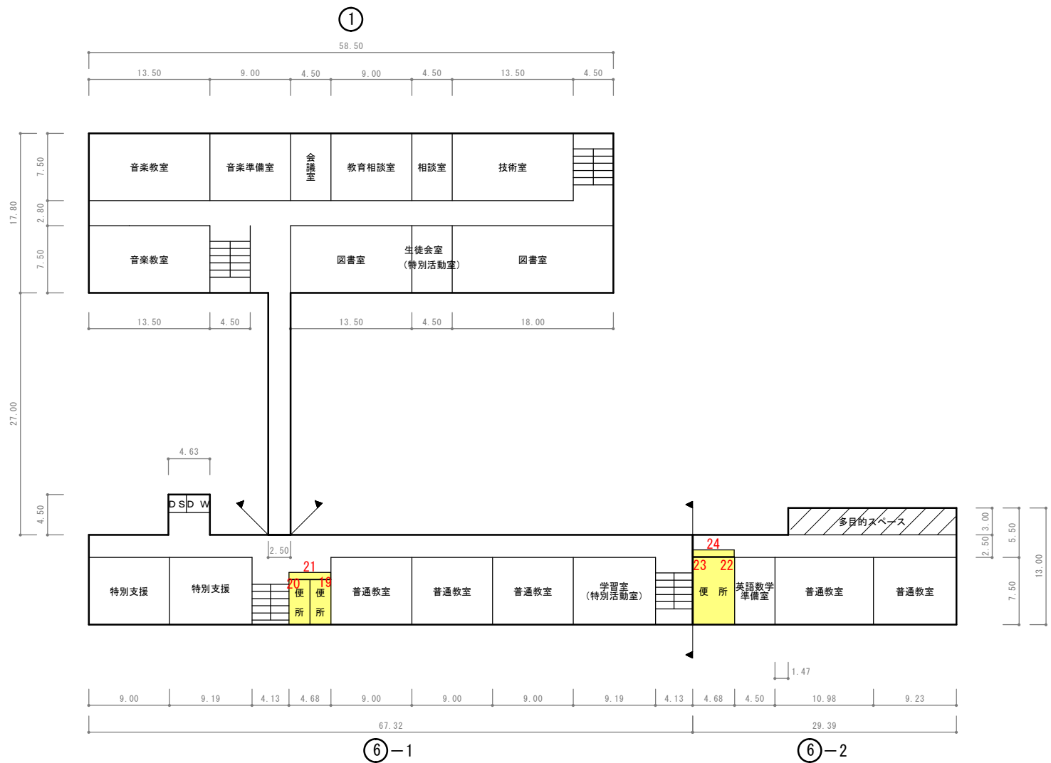
3 階 平 面 図
