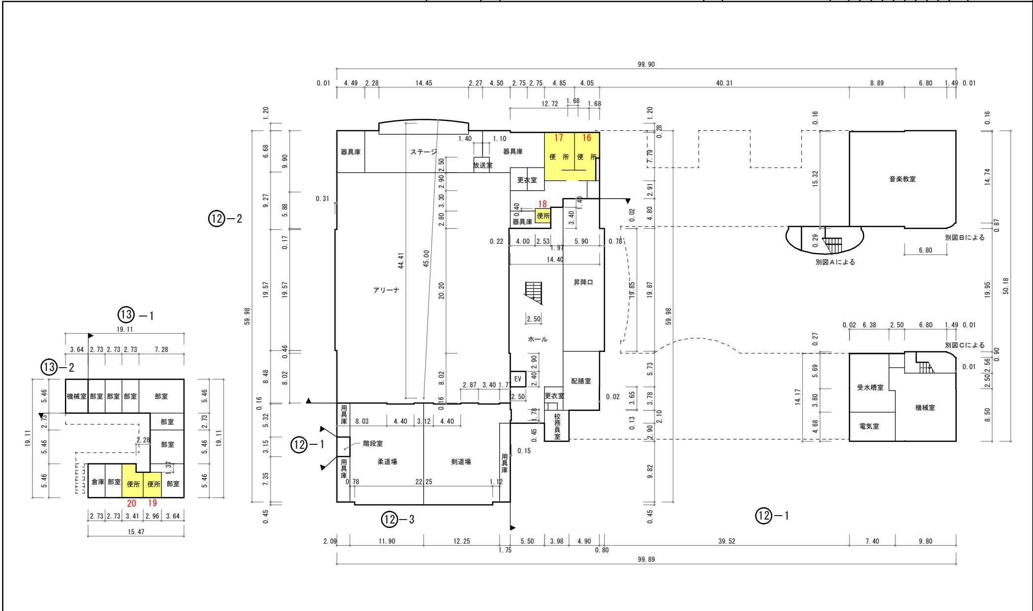
1 階 平 面 図
