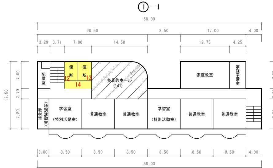
教室棟3階平面図
