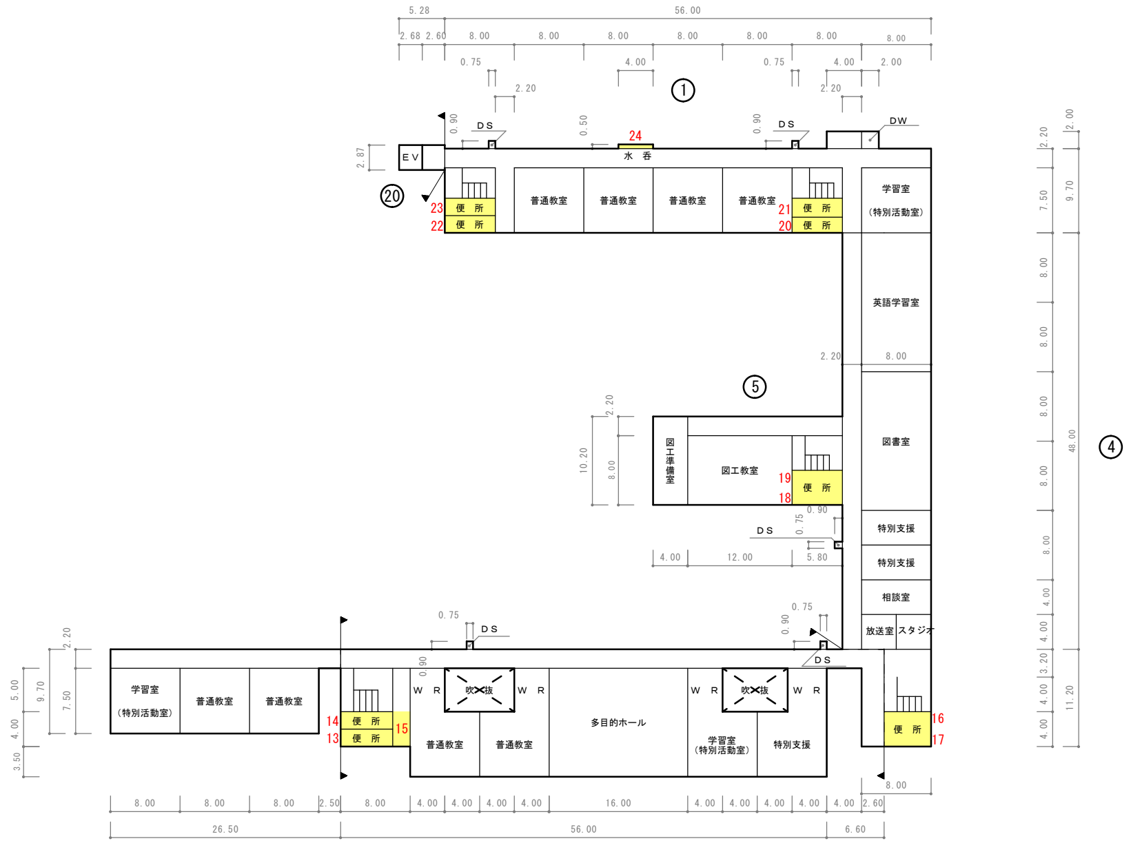
2階平面図
