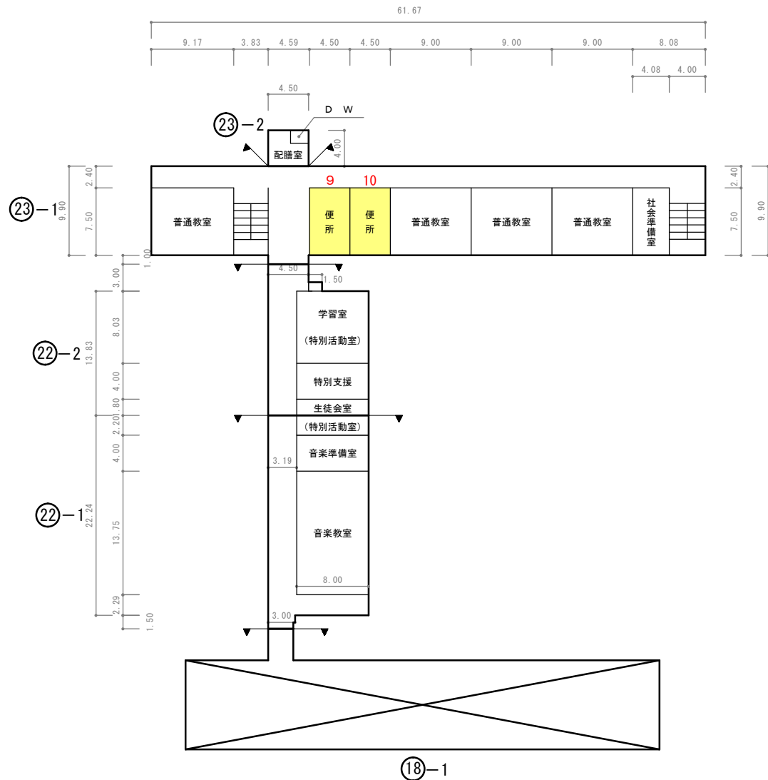
4 階 平面 図
