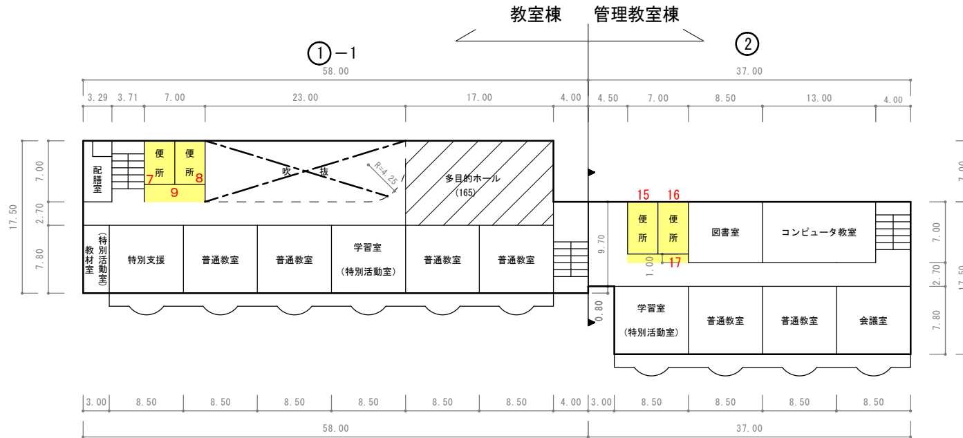
教室棟 2階平面図
