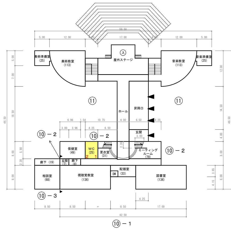
1階平面図
