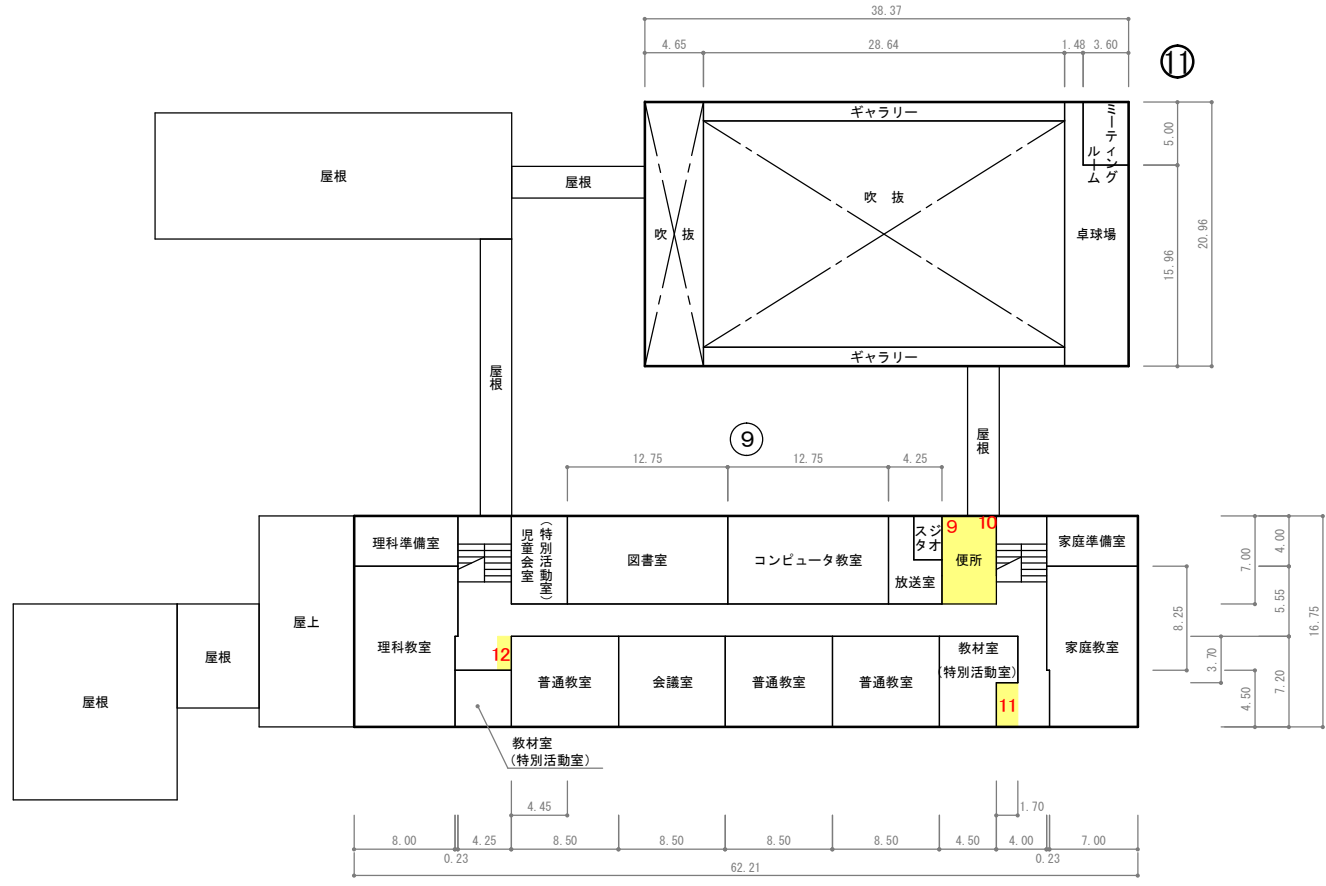
2階平面図
